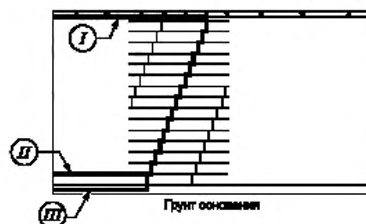
I — поступательный сдвиг по поверхности контакта между системой дорожной одежды и ППС; II — поступательный сдвиг смежных слоев ППС блоков; III — поступательный сдвиг по поверхности контакта ППС блоков и поверхности грунта основания
