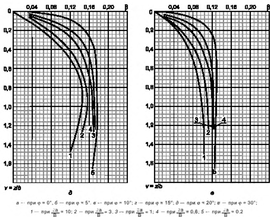
Рисунок В.17 — Графики для определения значения функции \beta
