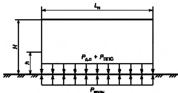
H — высота насыпи, м; h — уровень воды, м; L_n — ширина насыпи, м; P_{\text{воды}} — подъемная сила воды, кН/м; P_{\text{до}} — вес дорожной одежды, кН/м; P_{\text{ппс}} — вес насыпи из ППС блоков, кН/м
